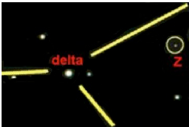
這張相片顯示北斗七星的特寫鏡頭，黃色概述大熊Z星位於大熊 \delta 星西北西星3度。
