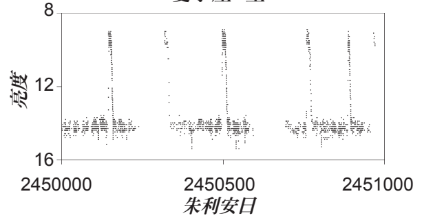
雙子座U星
