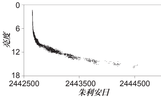
新星 - 天鵝V1500
